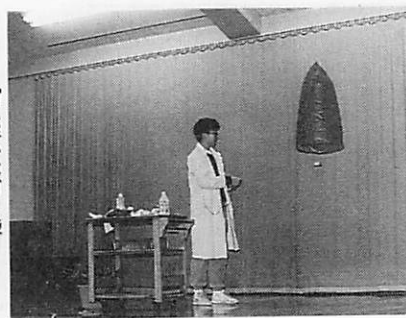
宙に浮かぶゴミ袋 — 理科の実験から —
